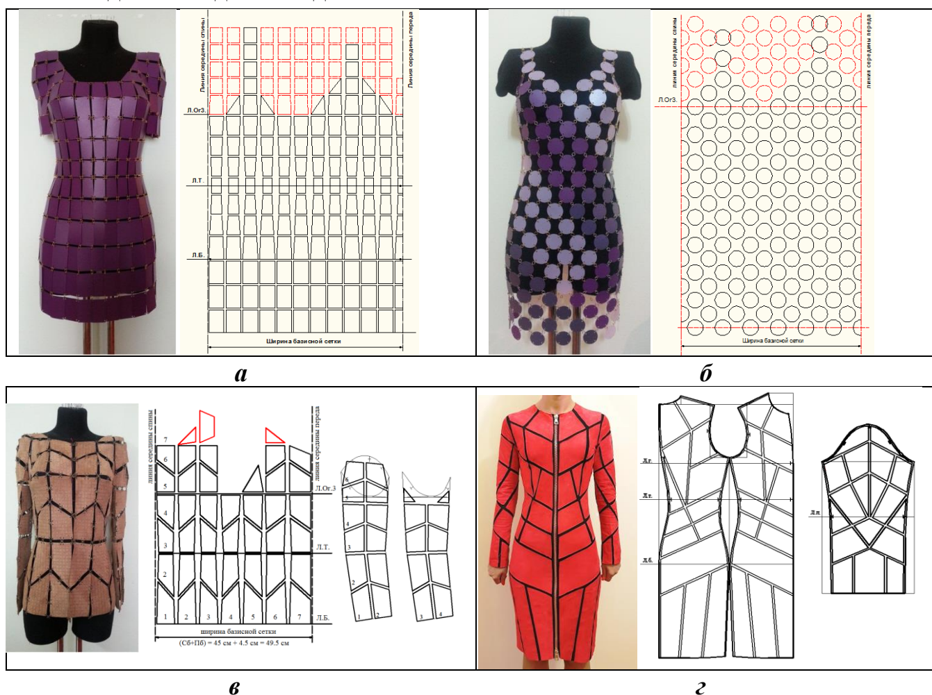
Рисунок 7 – Чертежи конструкций и внешний вид готовых мультидетальных изделий: женских однослойных платьев с неравными деталями кроя (а) и с равными деталями кроя (б), однослойного жакета из замши (в), двухслойного женского платья (г)
